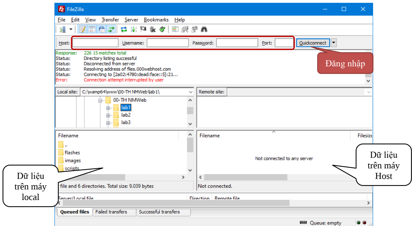
Giao diện chính của phần mềm hỗ trợ upload FileZilla
