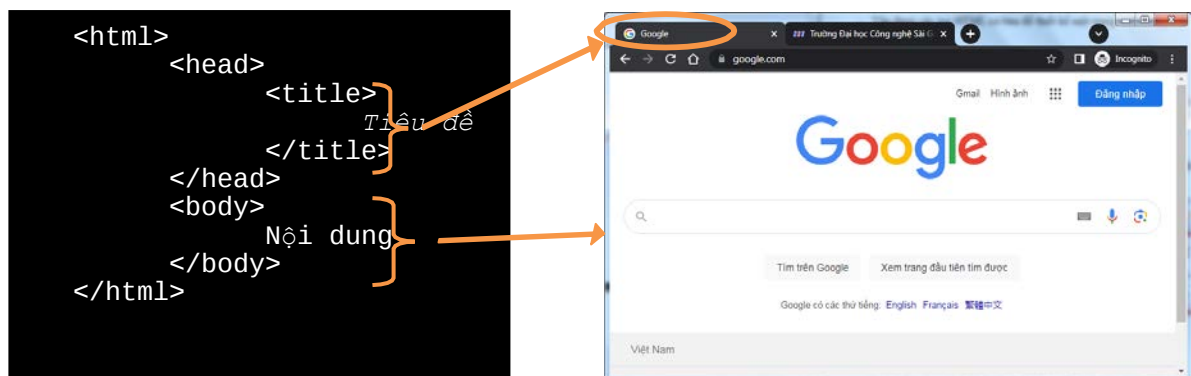
Hình 1.1: Cấu trúc cơ bản một trang HTML
